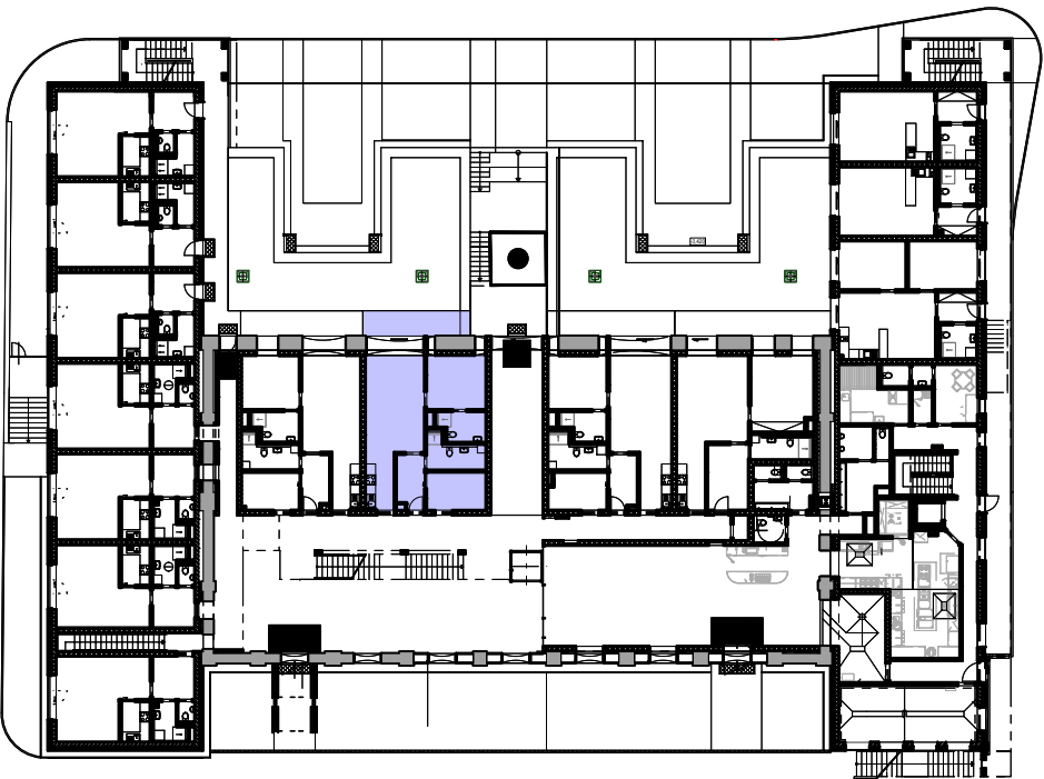
Schéma půdorys
